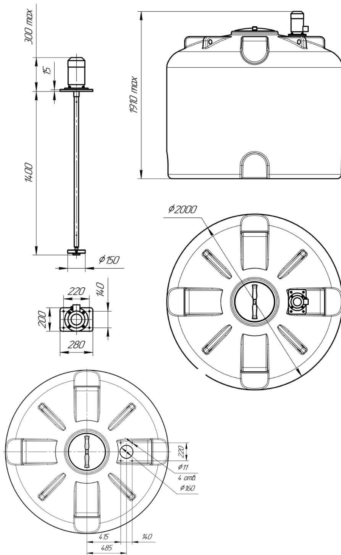
Габаритные размеры емкости TR 4500 с установленной мешалкой
