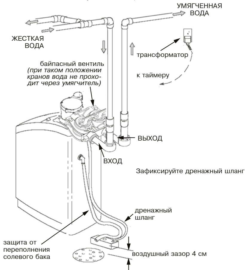
Рис. 4. Типовая схема установки
