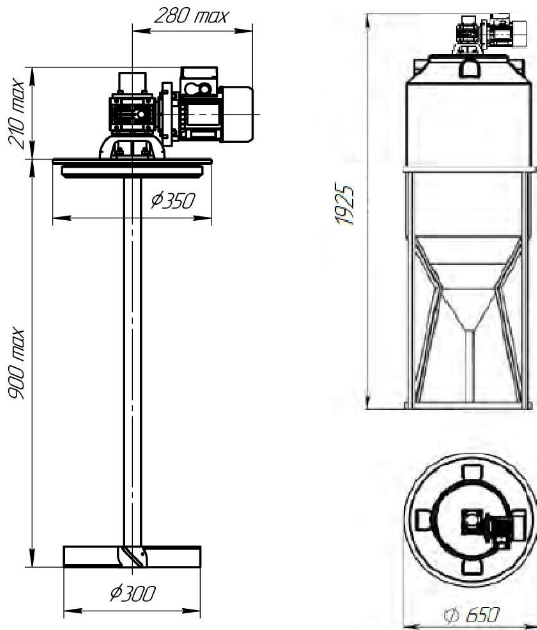
Габаритные размеры емкости ФМ 240 с установленной мешалкой
