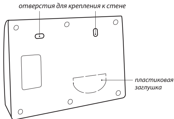
Рис. 7. Вид модуля управления Neptune ProW+ сзади
