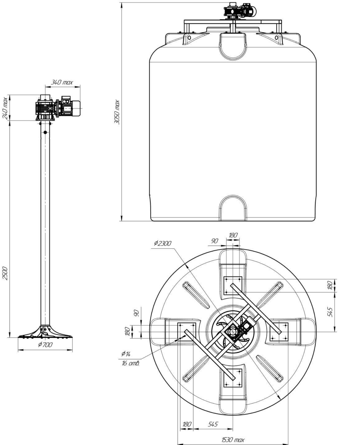
Габаритные размеры емкости TR10000 с установленной мешалкой
