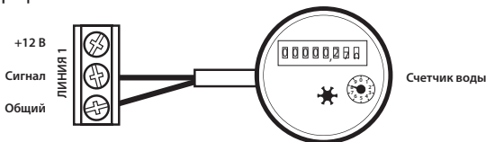
Рис. 3. Схема подключения прибора учета воды (счётчик) к модулю управления PROW+WiFi.
