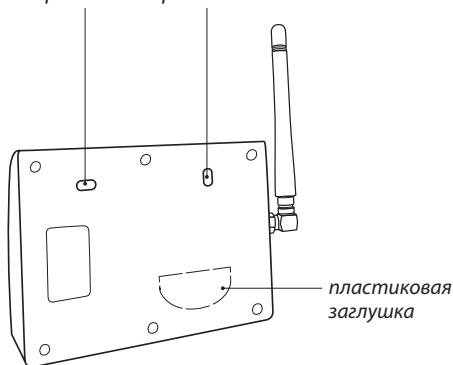
Рис. 7. Вид модуля управления Neptun ProW+ WiFi сзади
