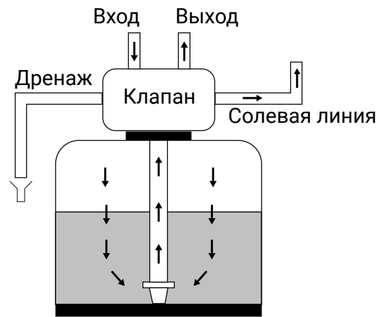
Заполнение бака-солеорастворителя
