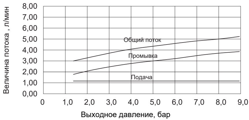
Инжектор 1 (Белый)
