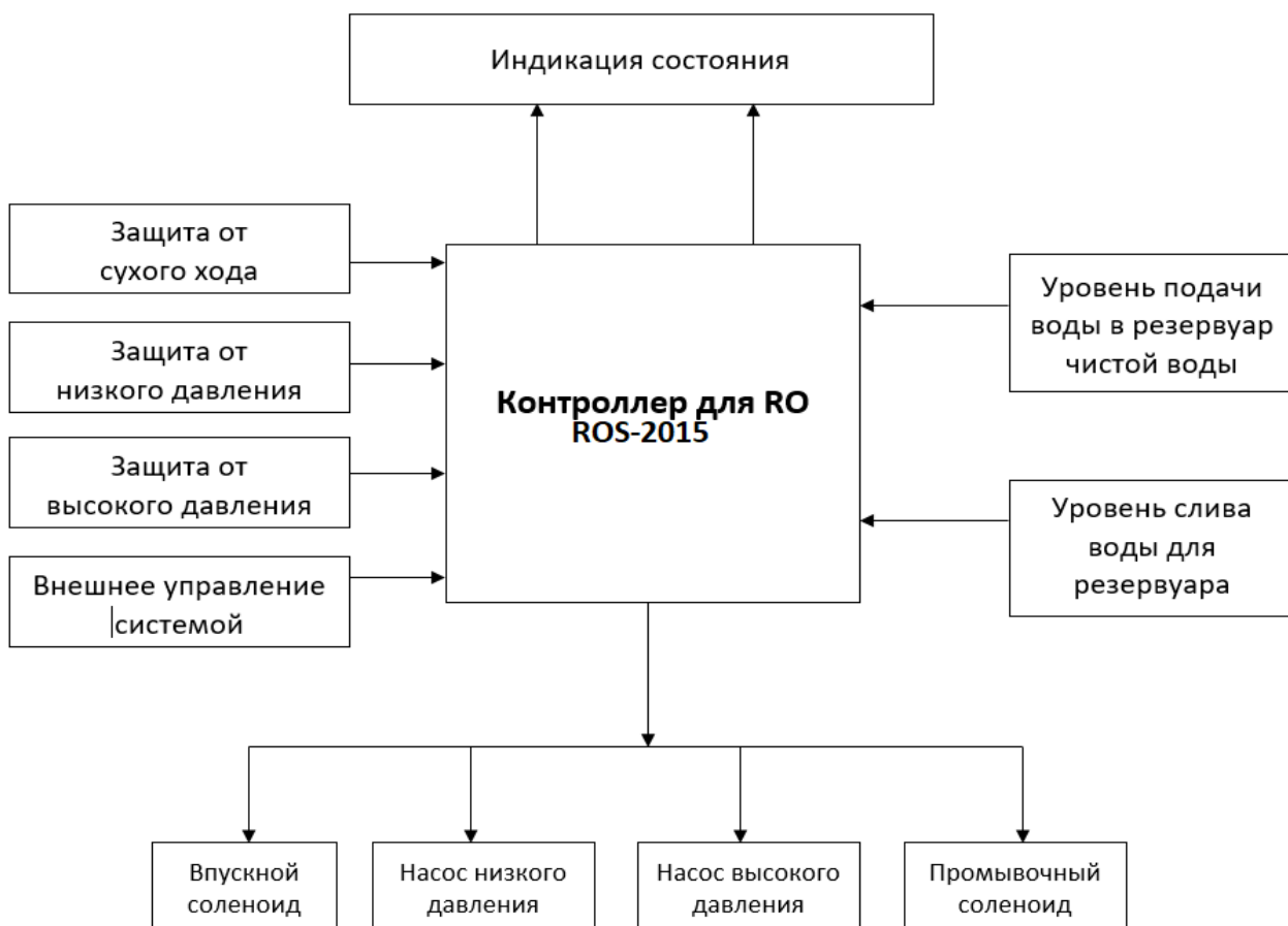
Рис. 1 Схема работы
