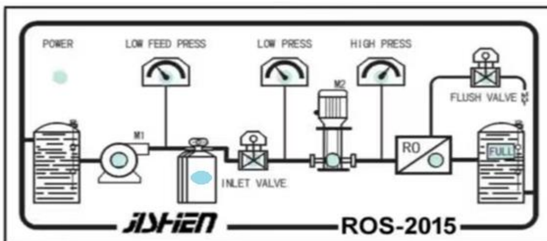
Рис.3 Панель дисплея
