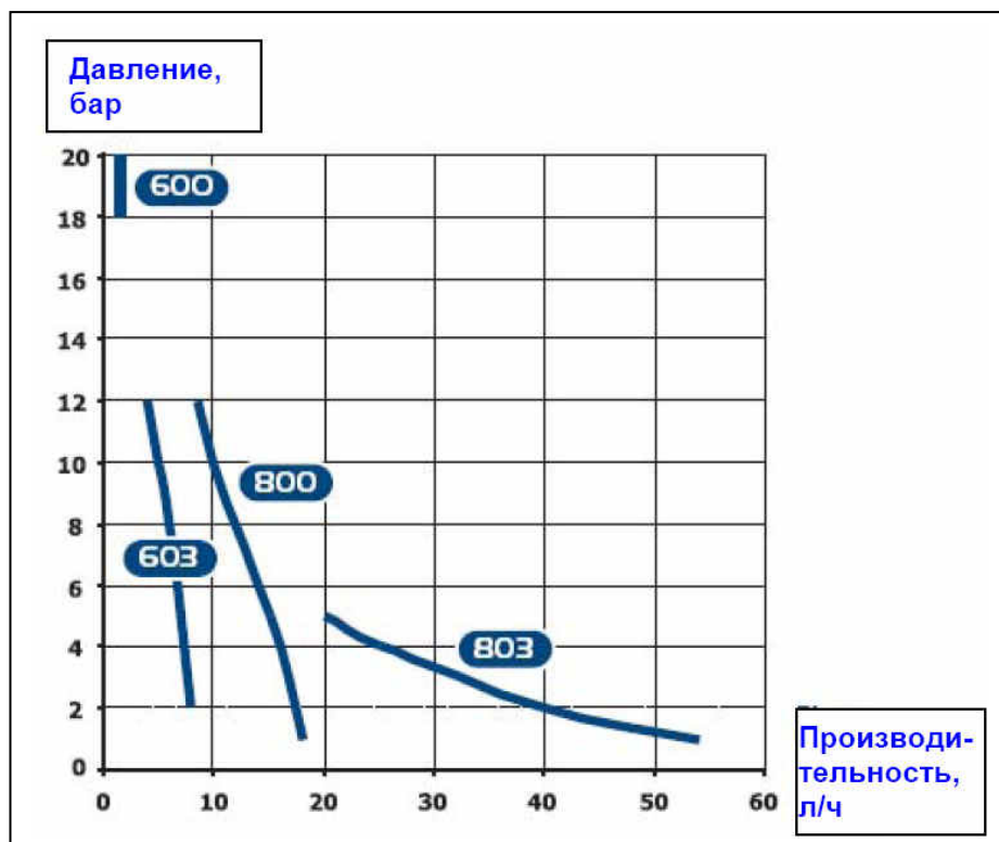
Рисунок 1. Диаграмма рабочих характеристик насосов-дозаторов
