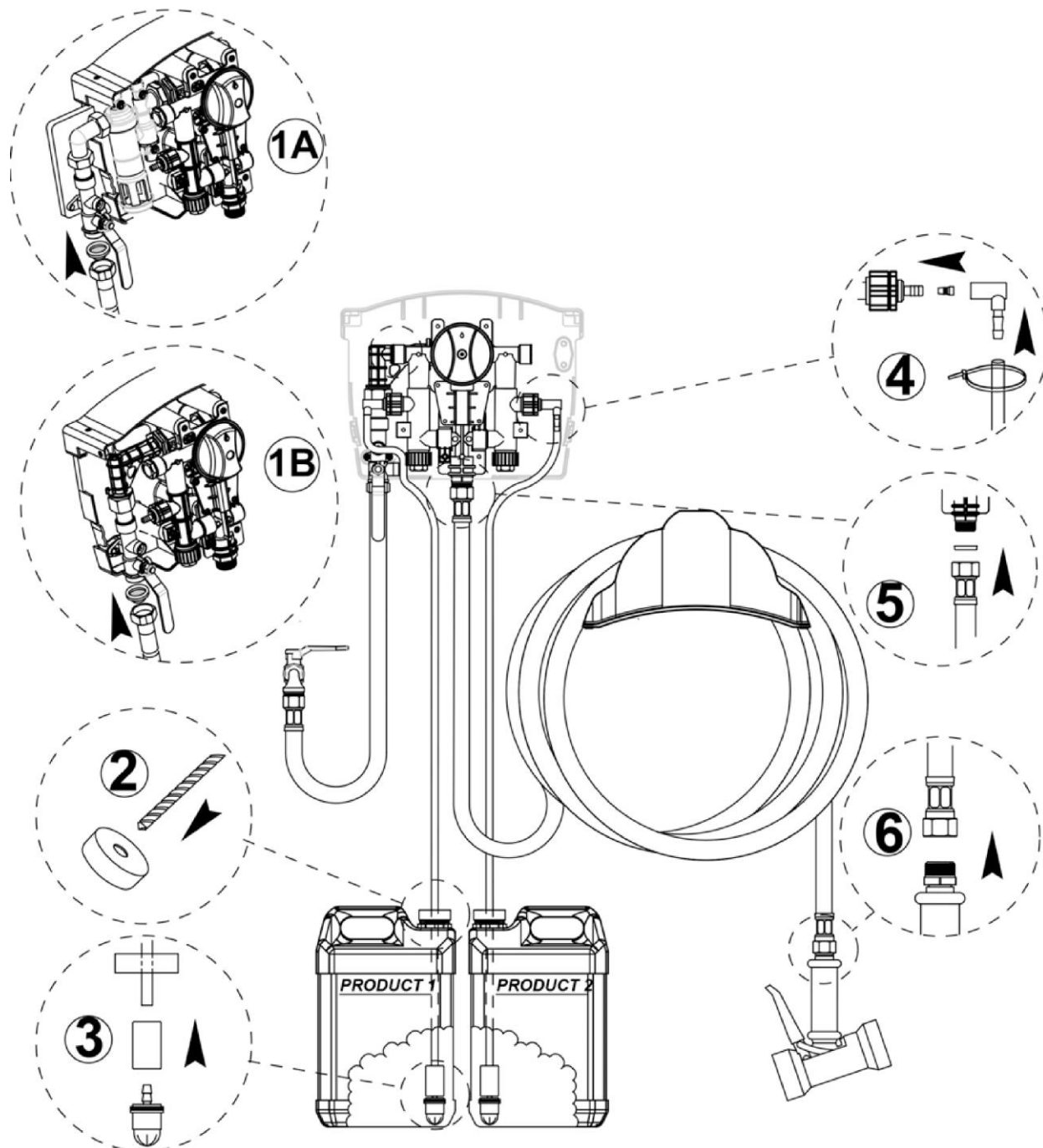
Рисунок 3 – установка
