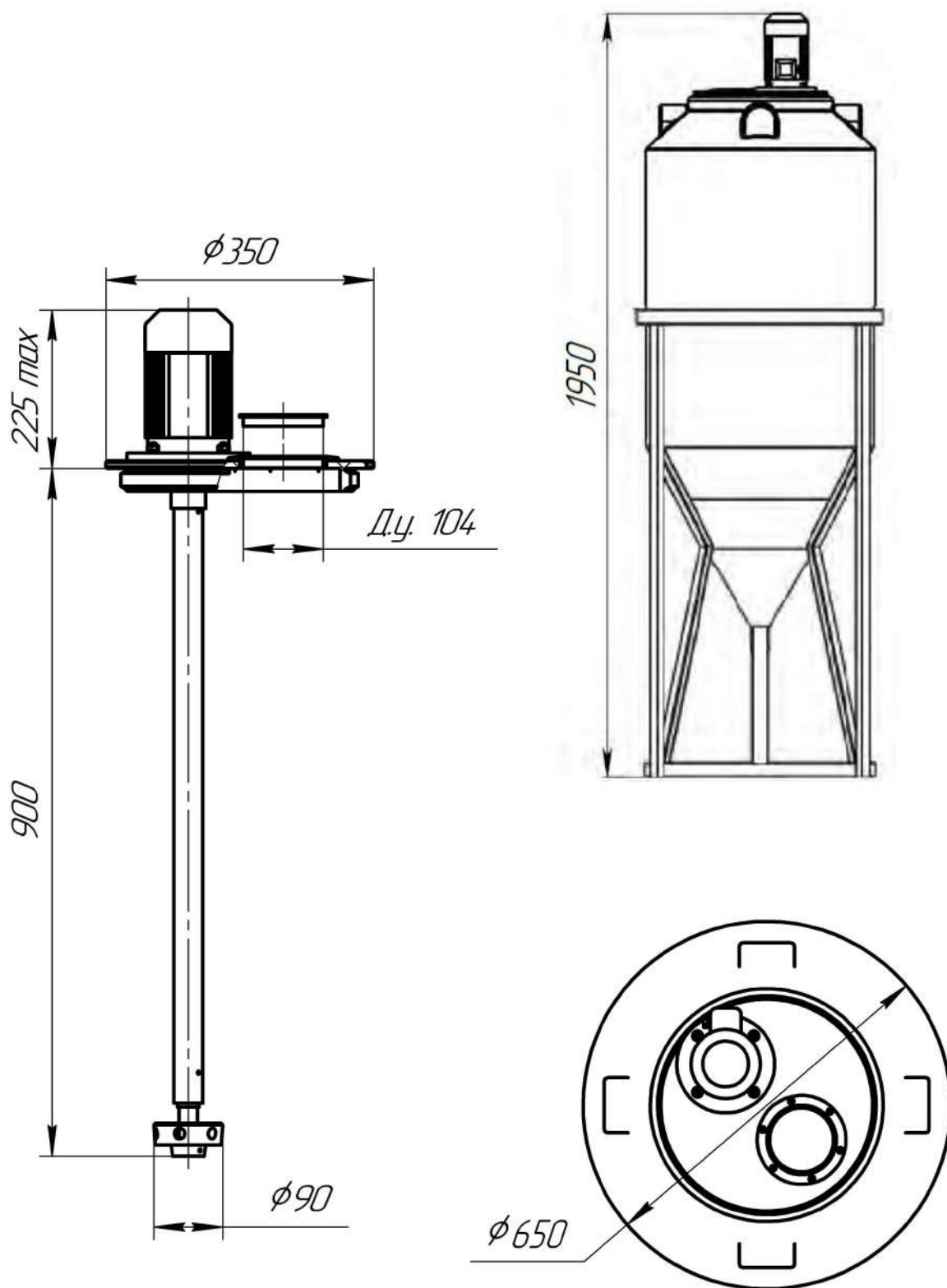
Габаритные размеры емкости ФМ 240 с установленной мешалкой
