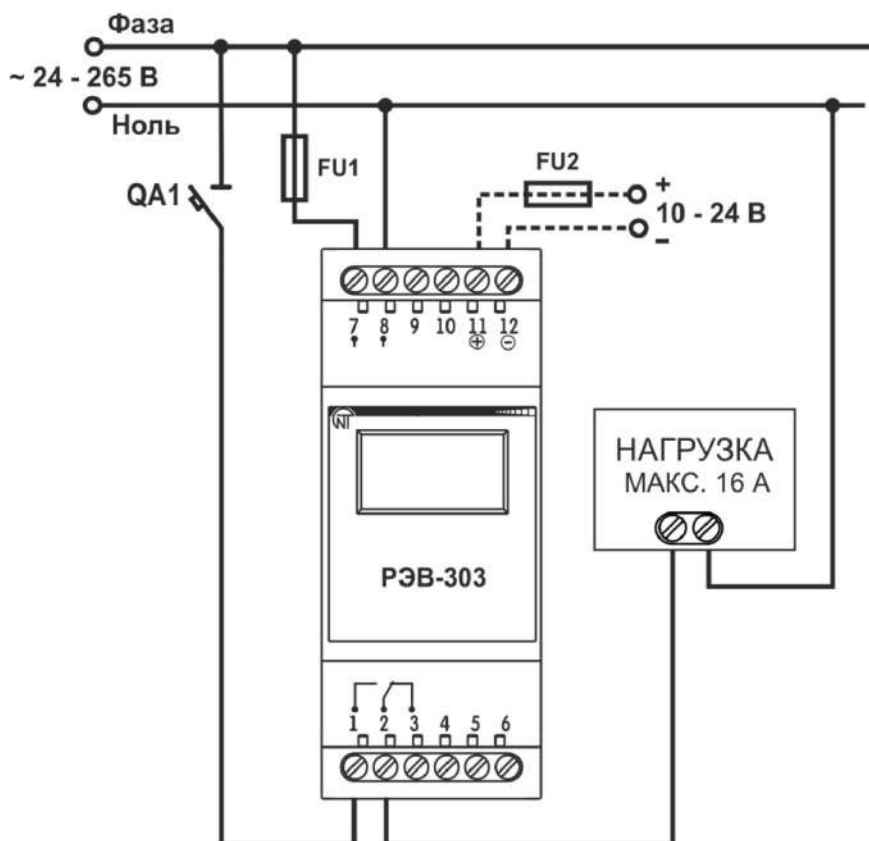
Рисунок 5.1 – Схема подключения РЭВ-303
