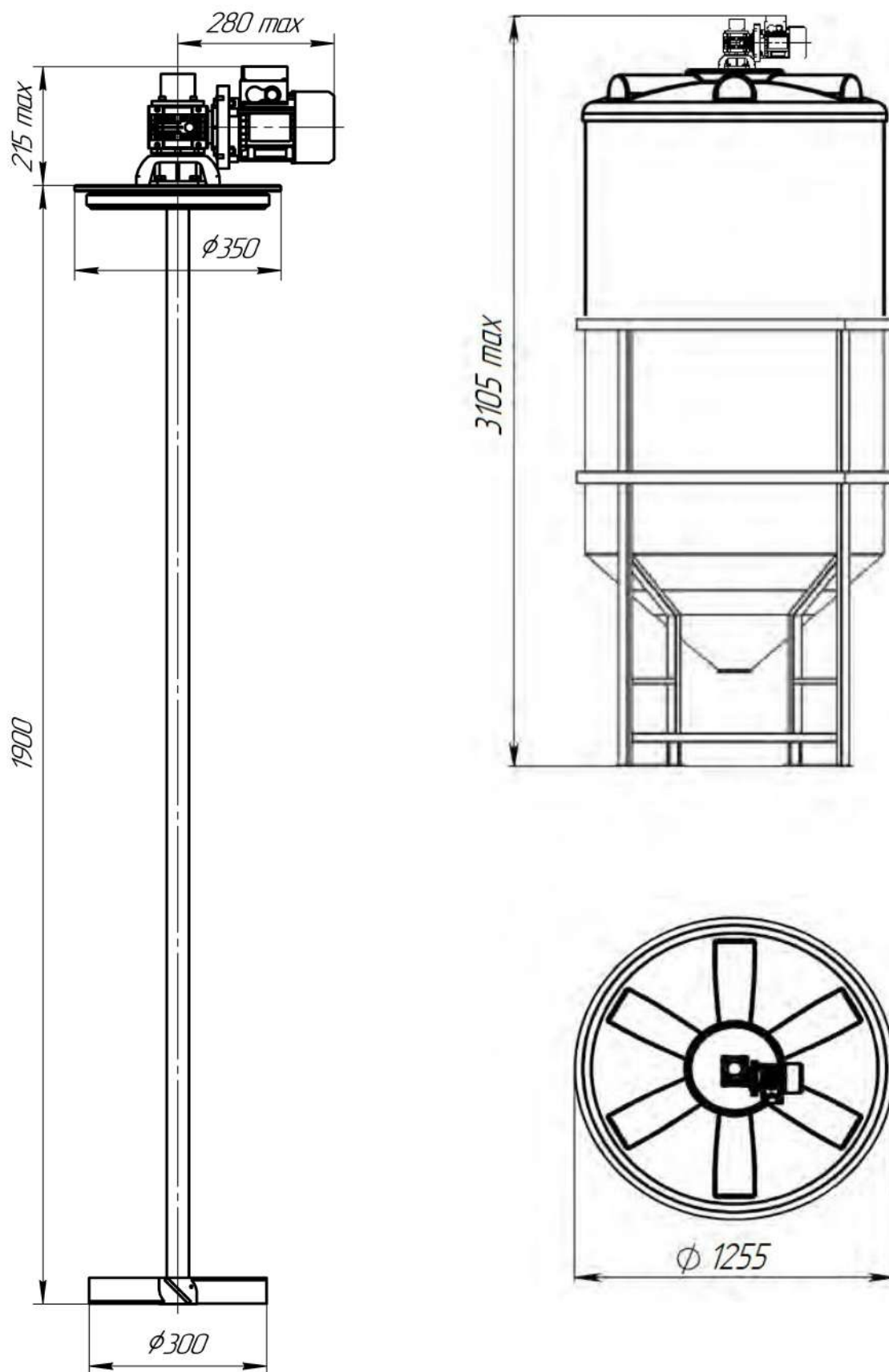
Габаритные размеры емкости ФМ 2000 с установленной мешалкой
