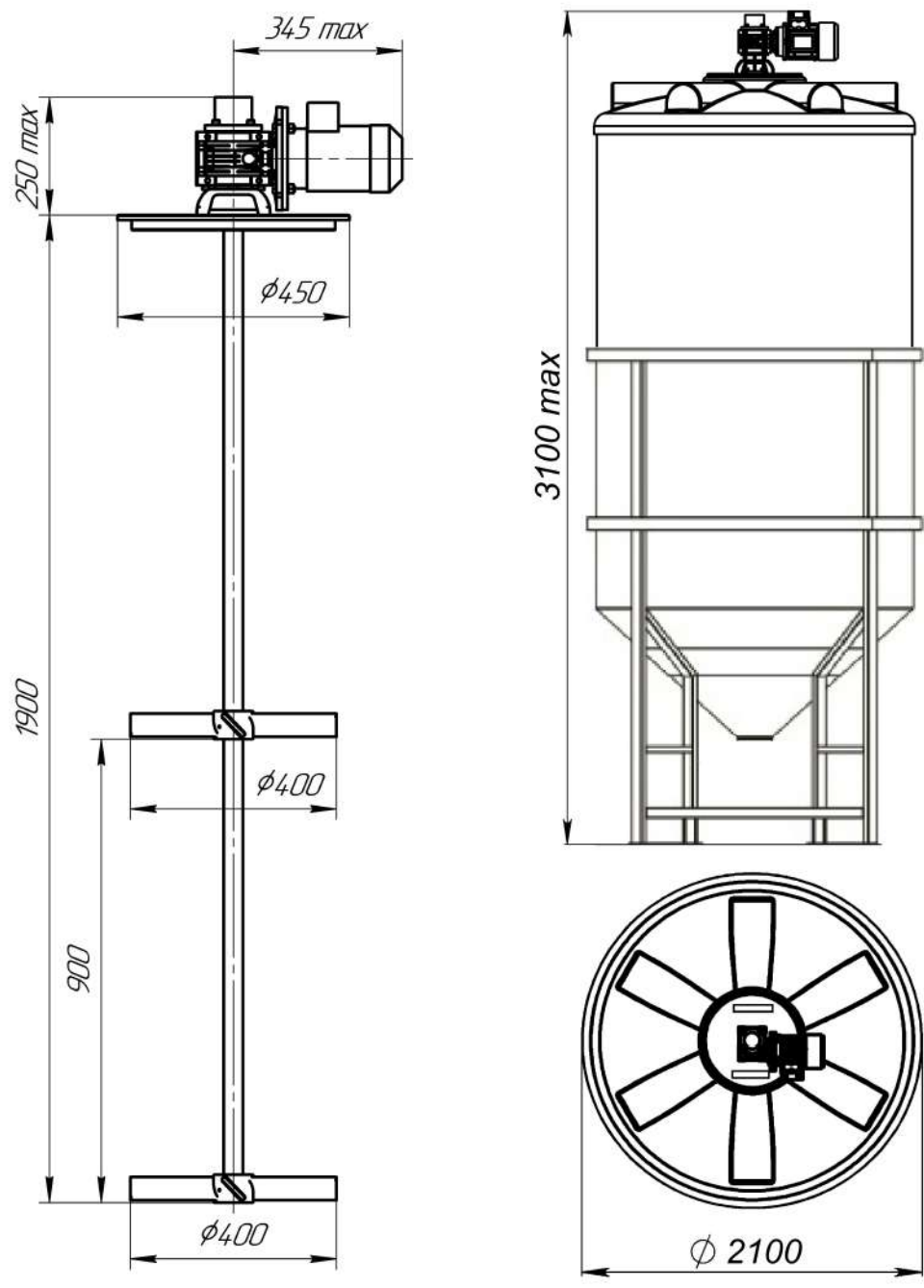
Габаритные размеры емкости ФМ 5000 с установленной мешалкой
