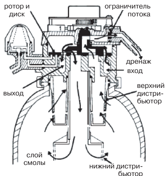
Рис. 11. Цикл обратной промывки
