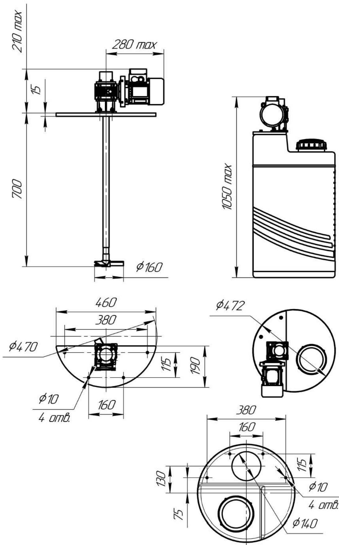
Габаритные размеры дозировочной ёмкости объёмом 100 литров с установленной мешалкой
