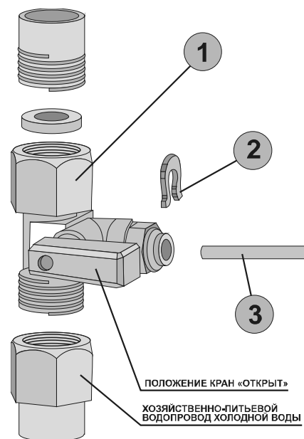
Рисунок 3. Узел подключения
