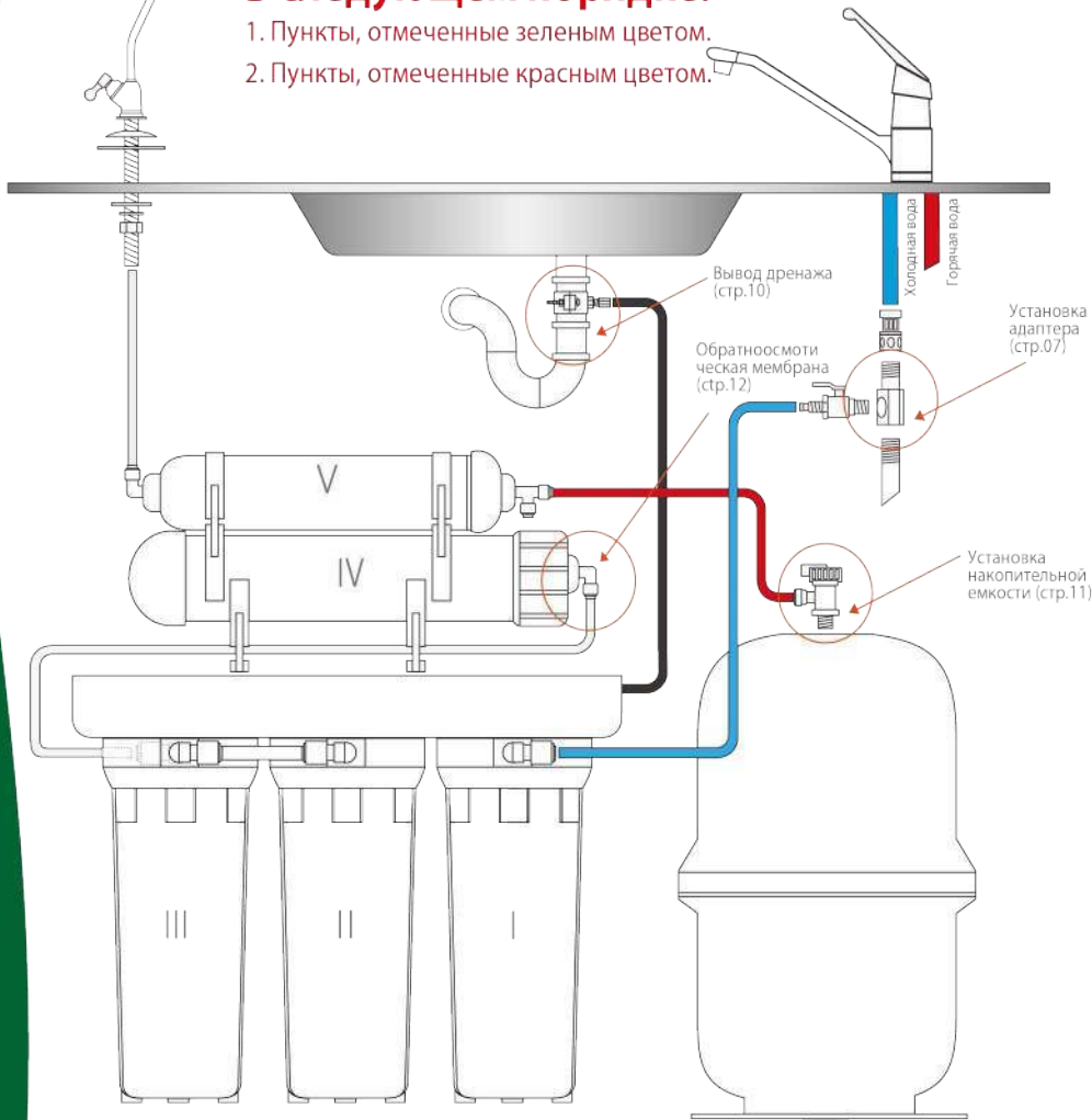
3 Соедините основной шаровой вентиль и адаптер
