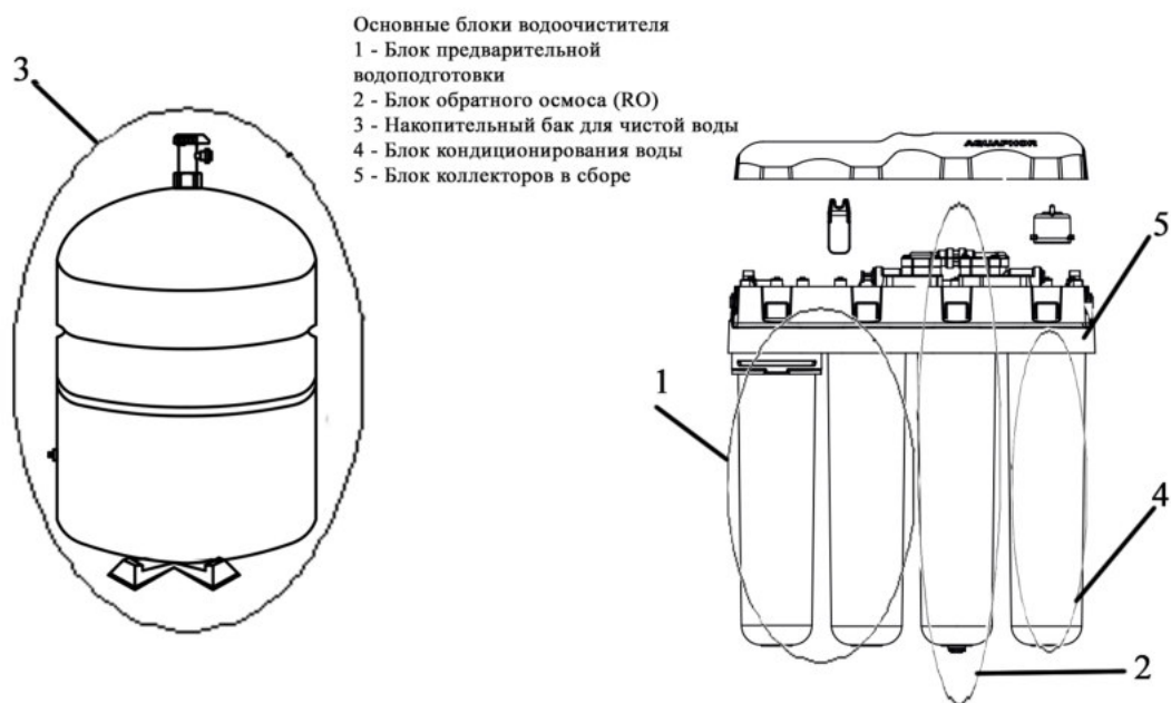
Рисунок 1. Устройство водоочистителя
