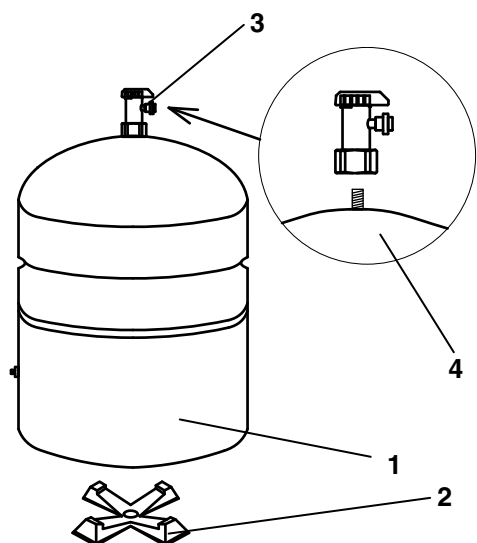
Рисунок 6. Накопительный бак
