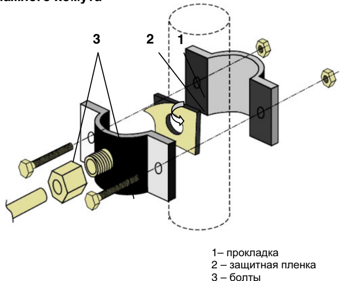
Рисунок 4. Дренажный хомут
