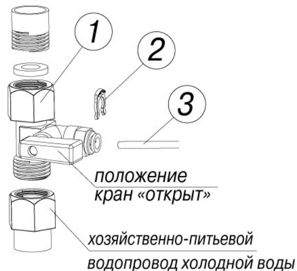
Рисунок 2. Узел подключения
