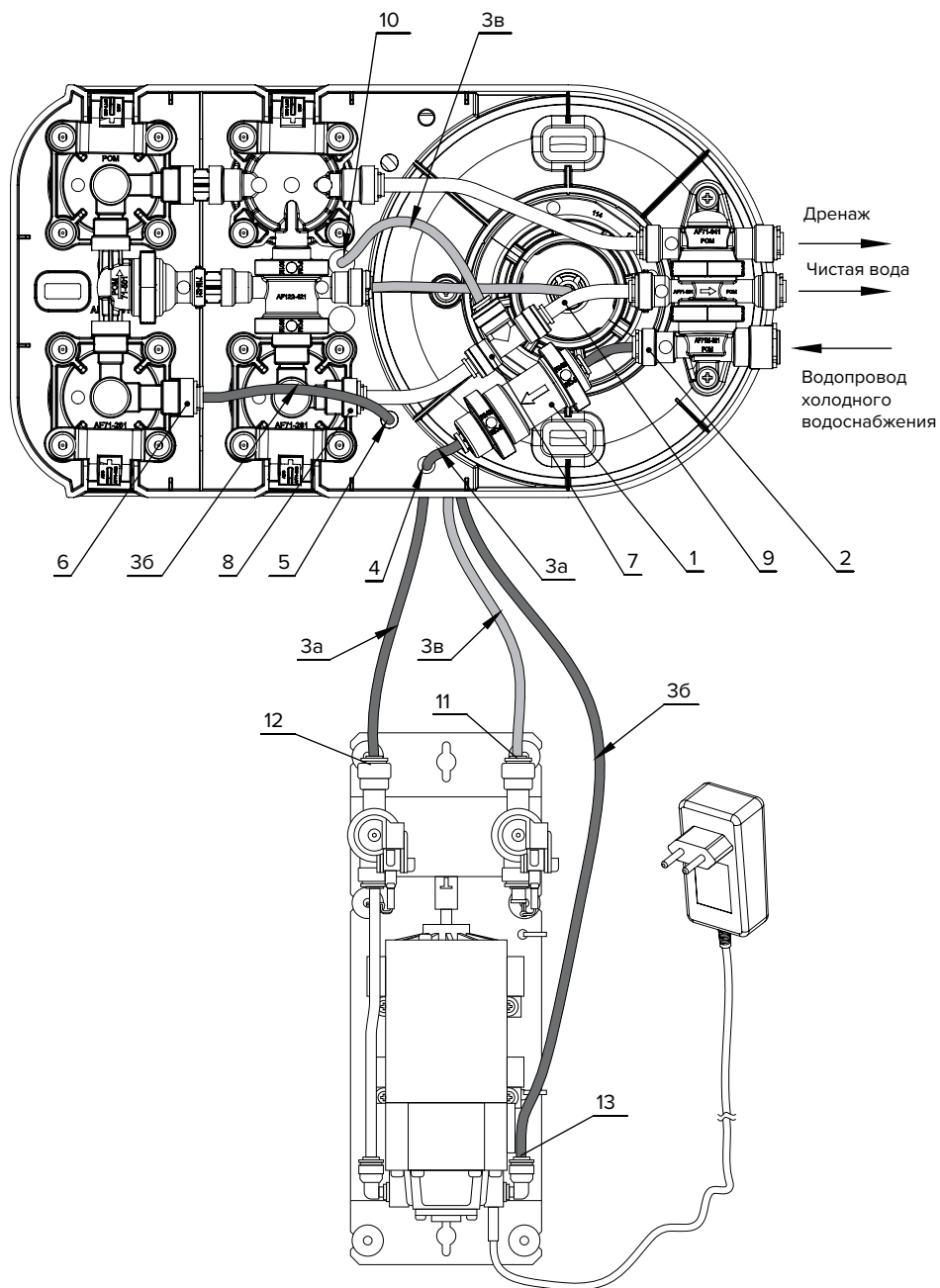
Рисунок 5. Схема подключения КПД к автоматам питьевой воды Аквафор Морион DWM-101S и DWM-101
