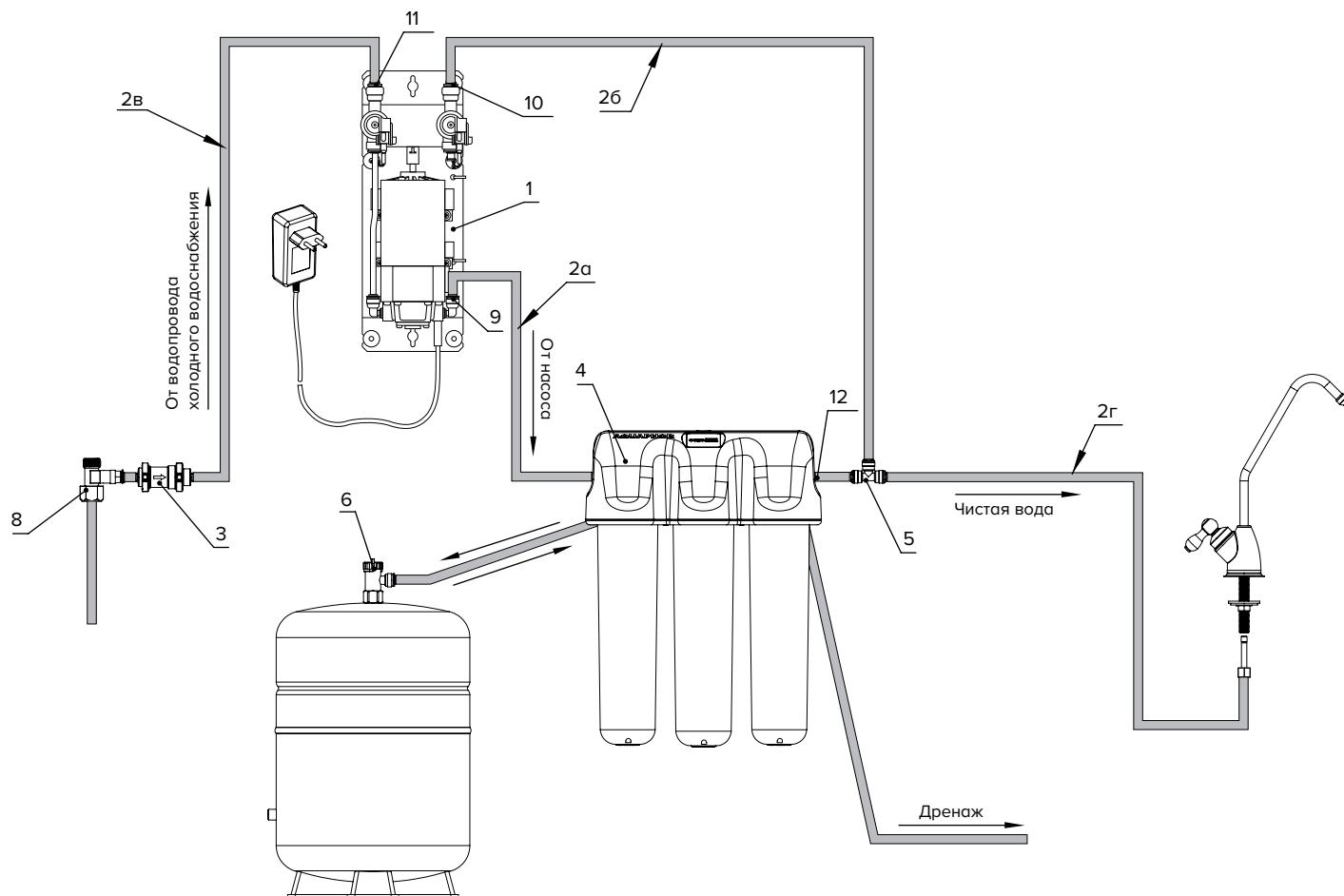
Рисунок 8. Схема подключения КПД водоочистителю Аквафор OSMO Pro 50 (OSMO Pro 100)
