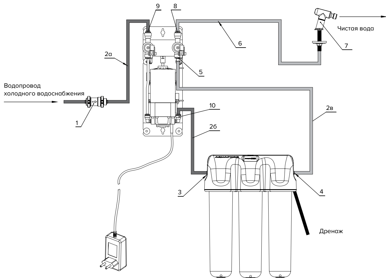
Рисунок 7. Схема подключения КПД к автомату питьевой воды Аквафор DWM-312S Pro
